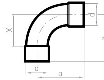
Bend 90° - FF
