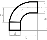
Bend 90° - FF
