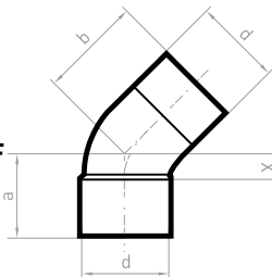
Elbow 45° - MF
