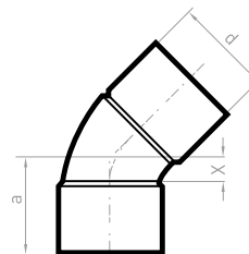
Elbow 45° - FF
